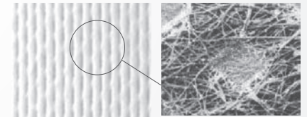
Fig.04 (surface soudée par point) Zoom soudure par point
