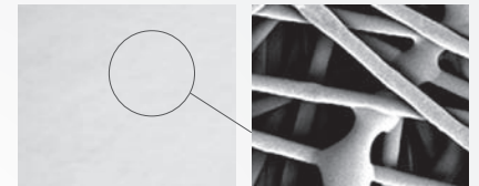
Fig.02 (surface lisse) Zoom soudure thermique
